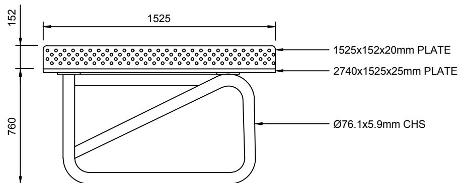
END ELEVATION
