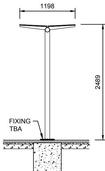
END ELEVATION
