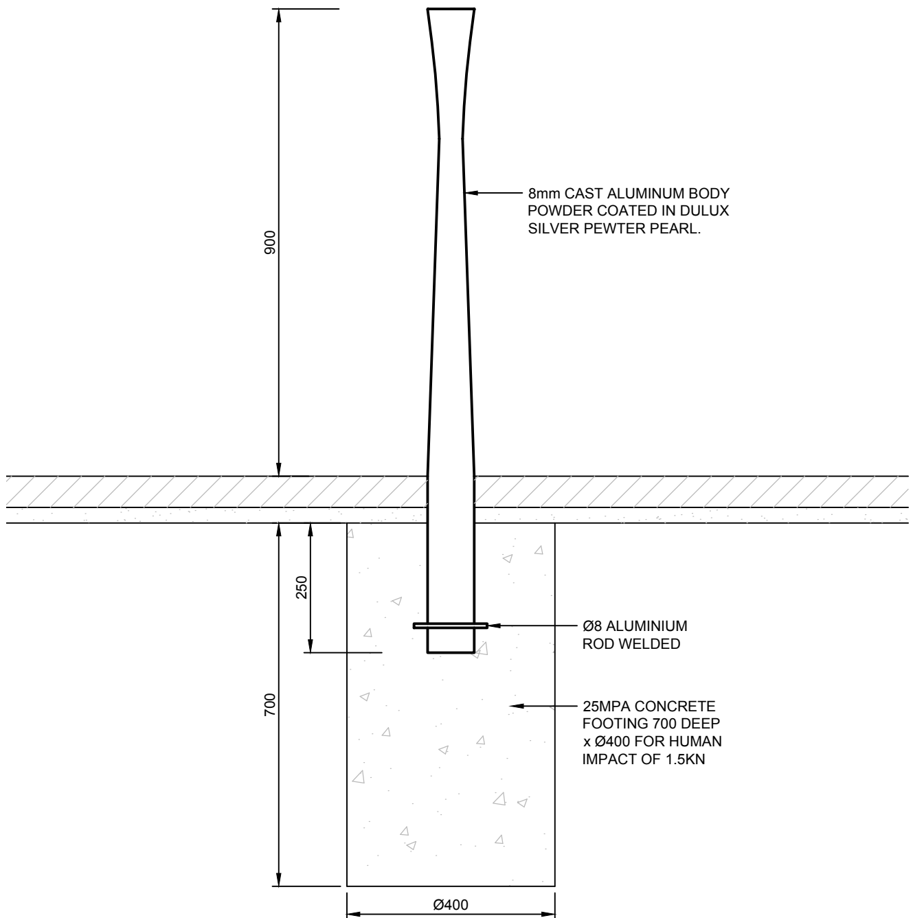
ELEVATION
