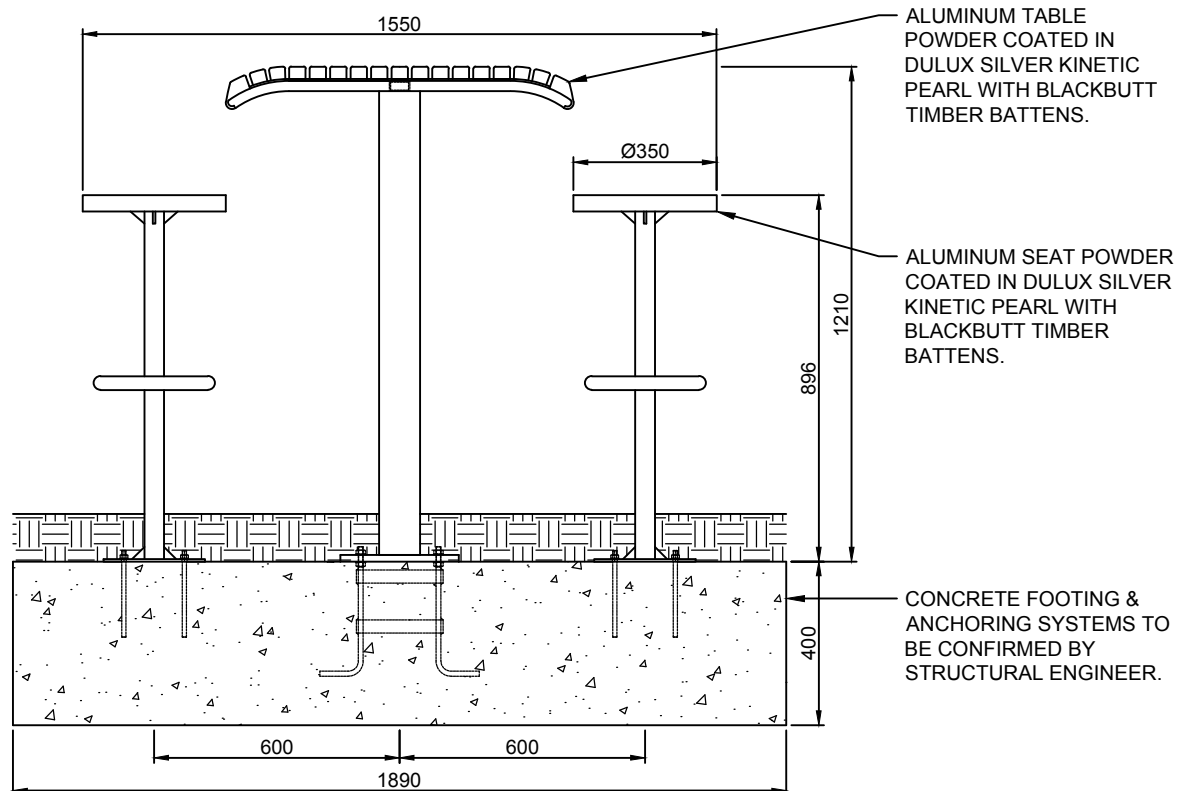
END ELEVATION
