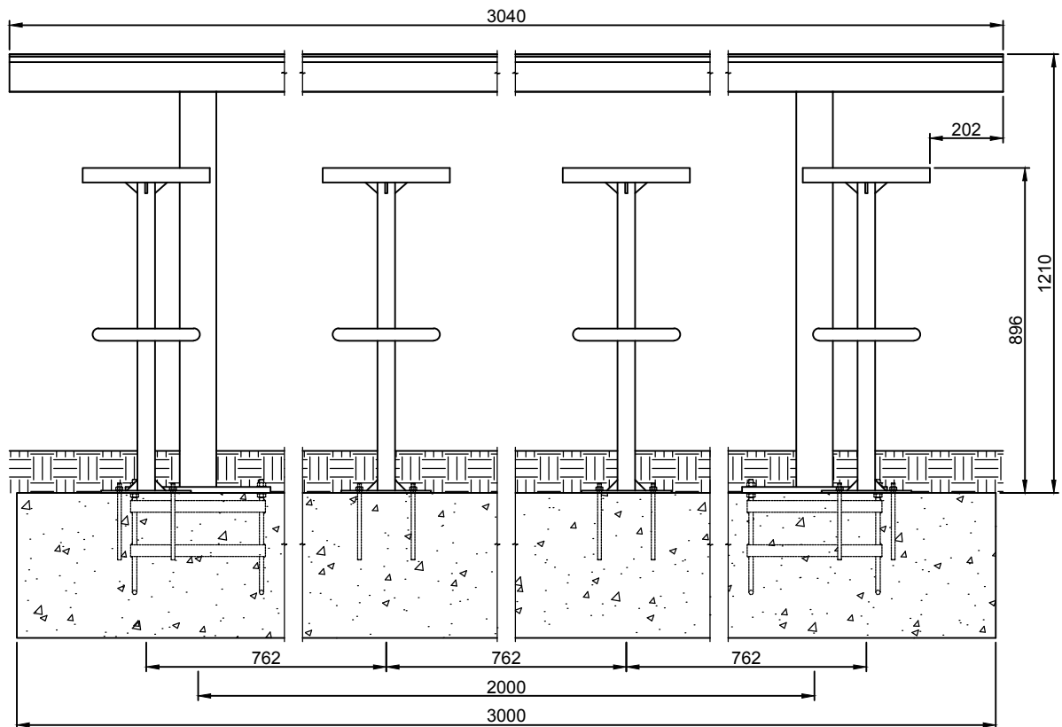
ELEVATION
