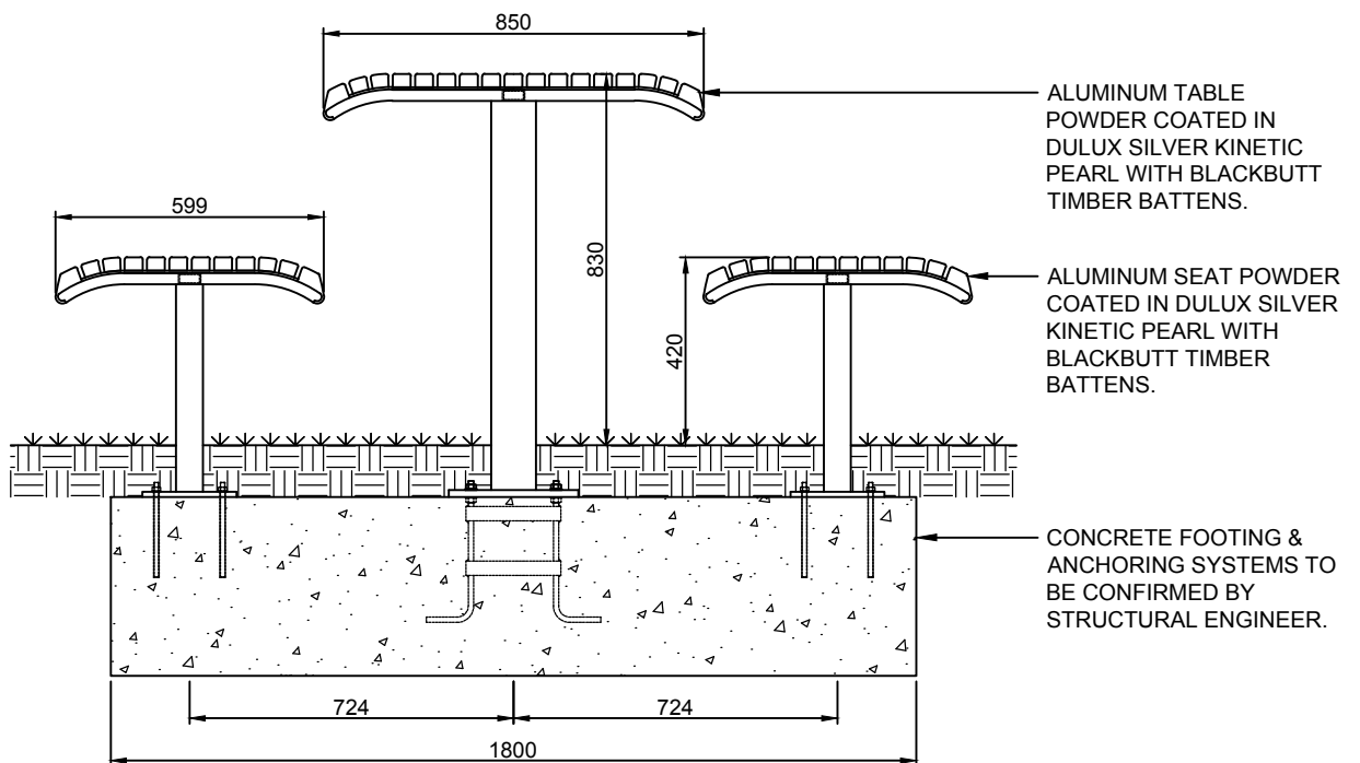
END ELEVATION
