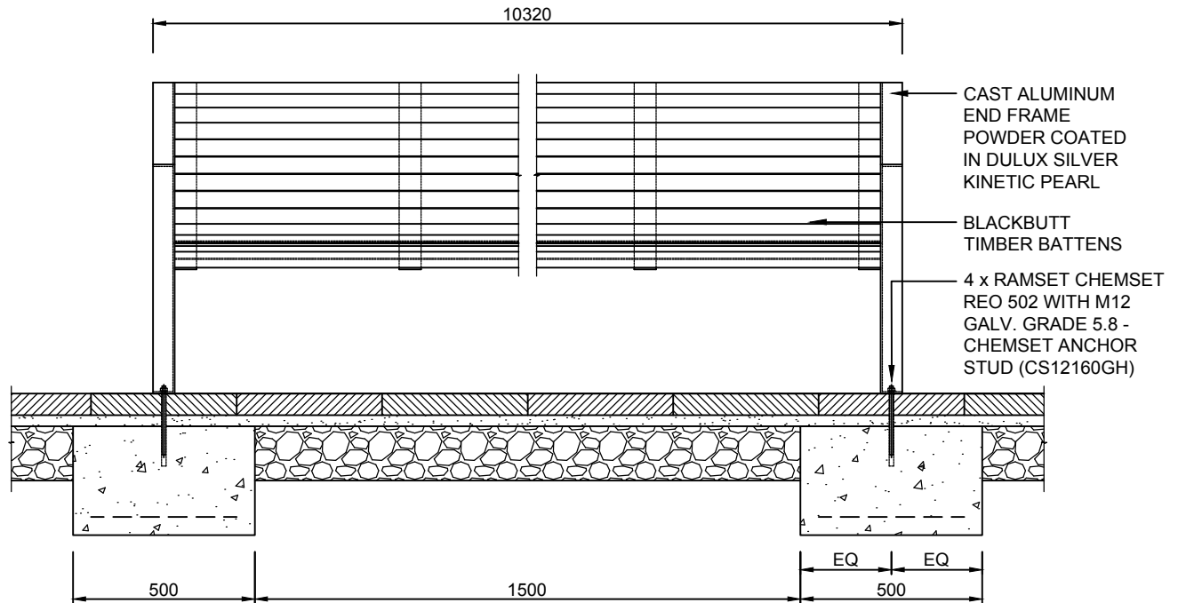
ELEVATION
