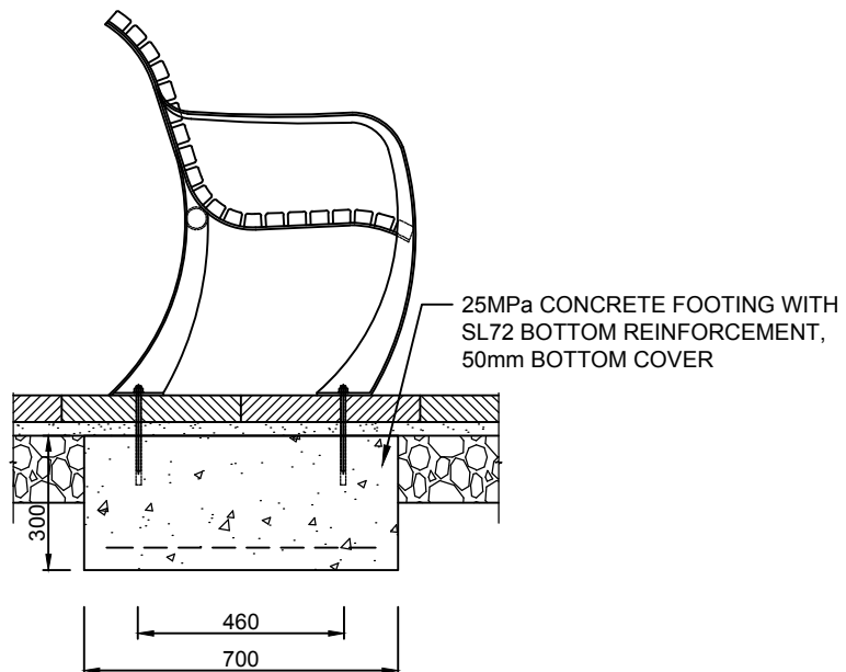
END ELEVATION
