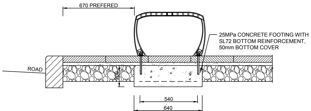
END ELEVATION
