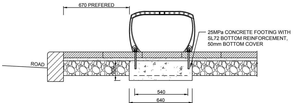
END ELEVATION
