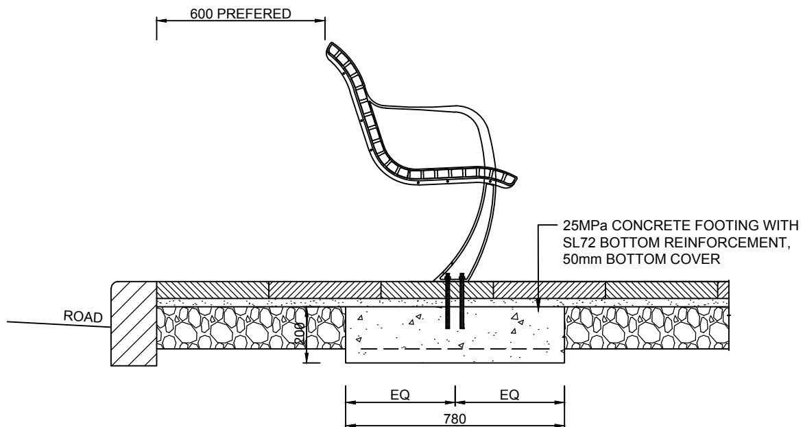
END ELEVATION
