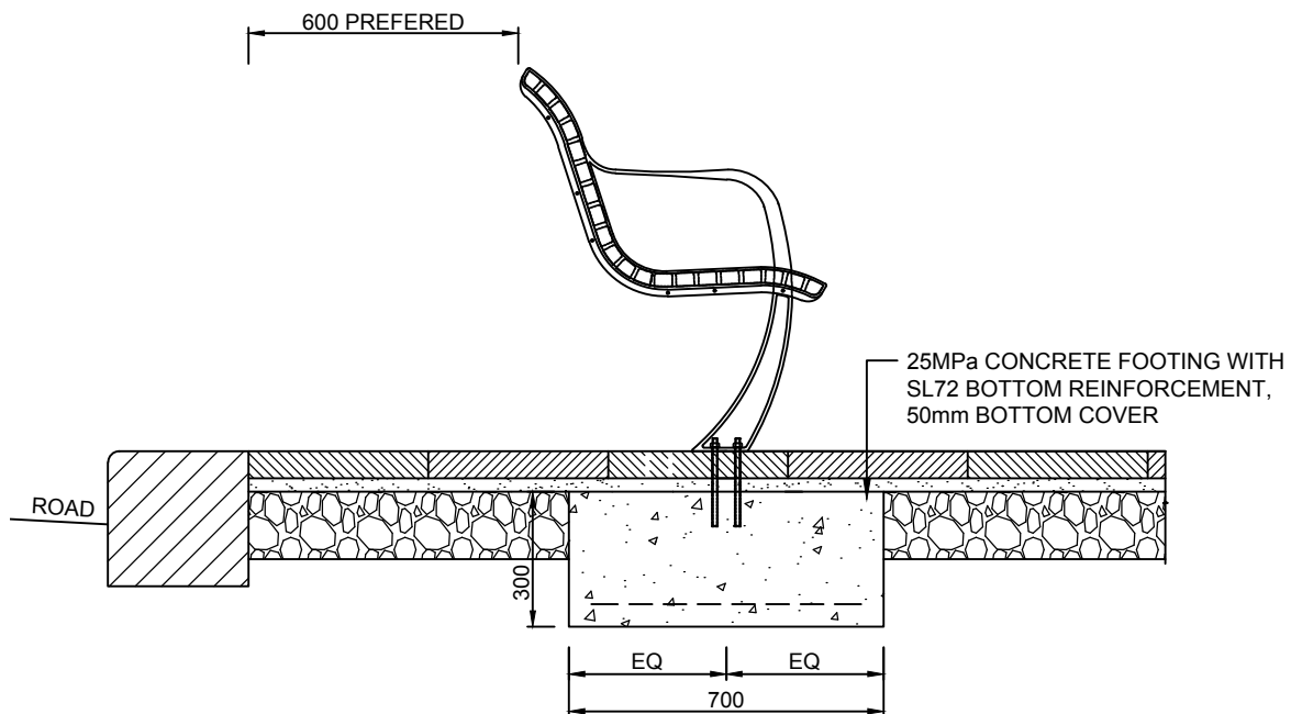
END ELEVATION
